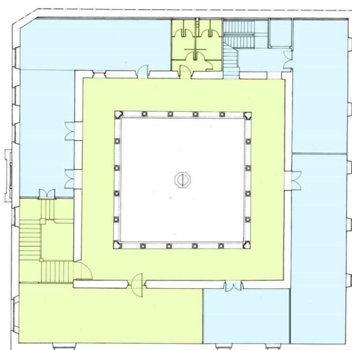
Planta N1
